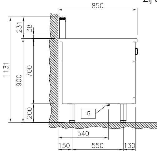
Zij aanzicht
